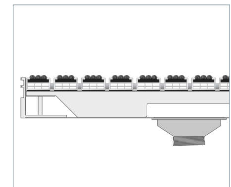
Querschnitt mit Ablauf
