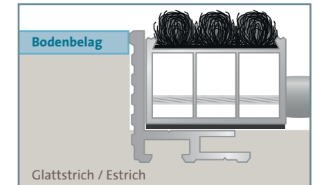
Montage: Der Winkelrahmen muss bündig mit Bodenbelag und Glattstrich / Estrich abschließen
